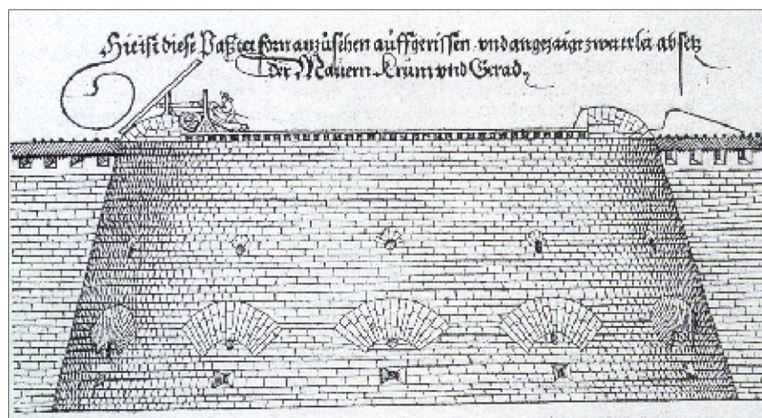
PARAPETO A BARBETA DEL TRATADO DE DURERO
